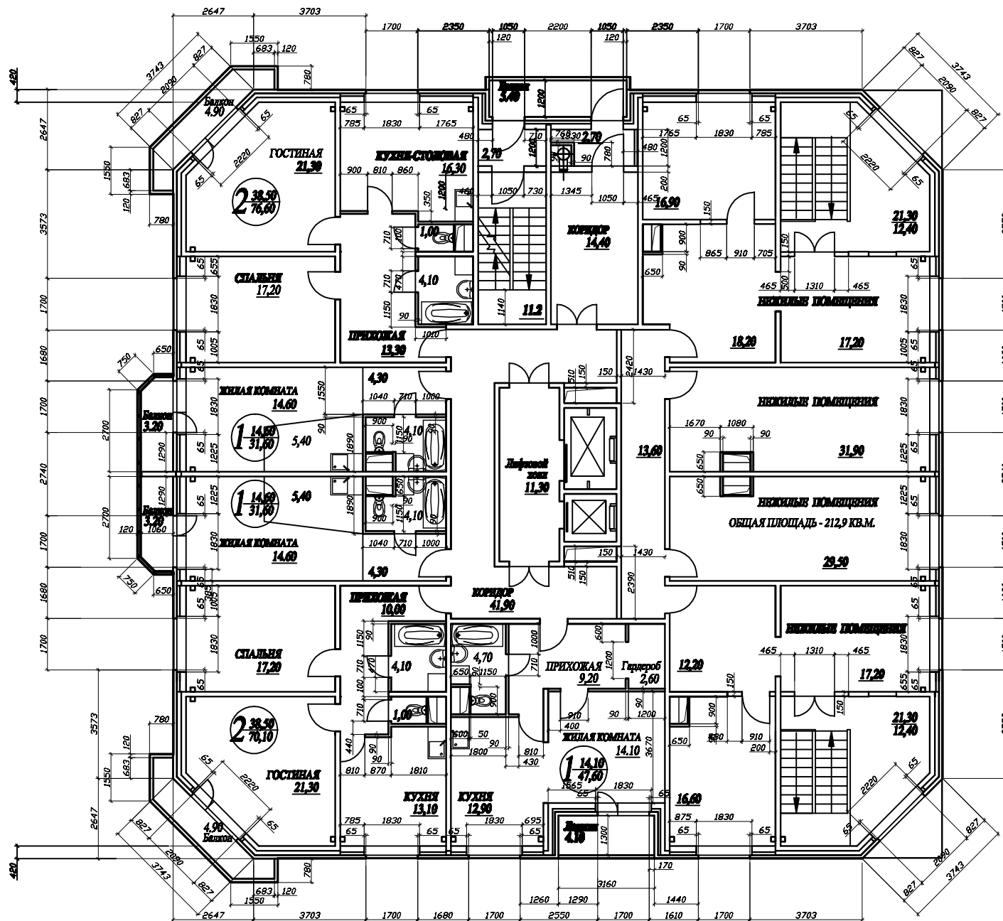
Корпус № 6 План 2-го этажа
