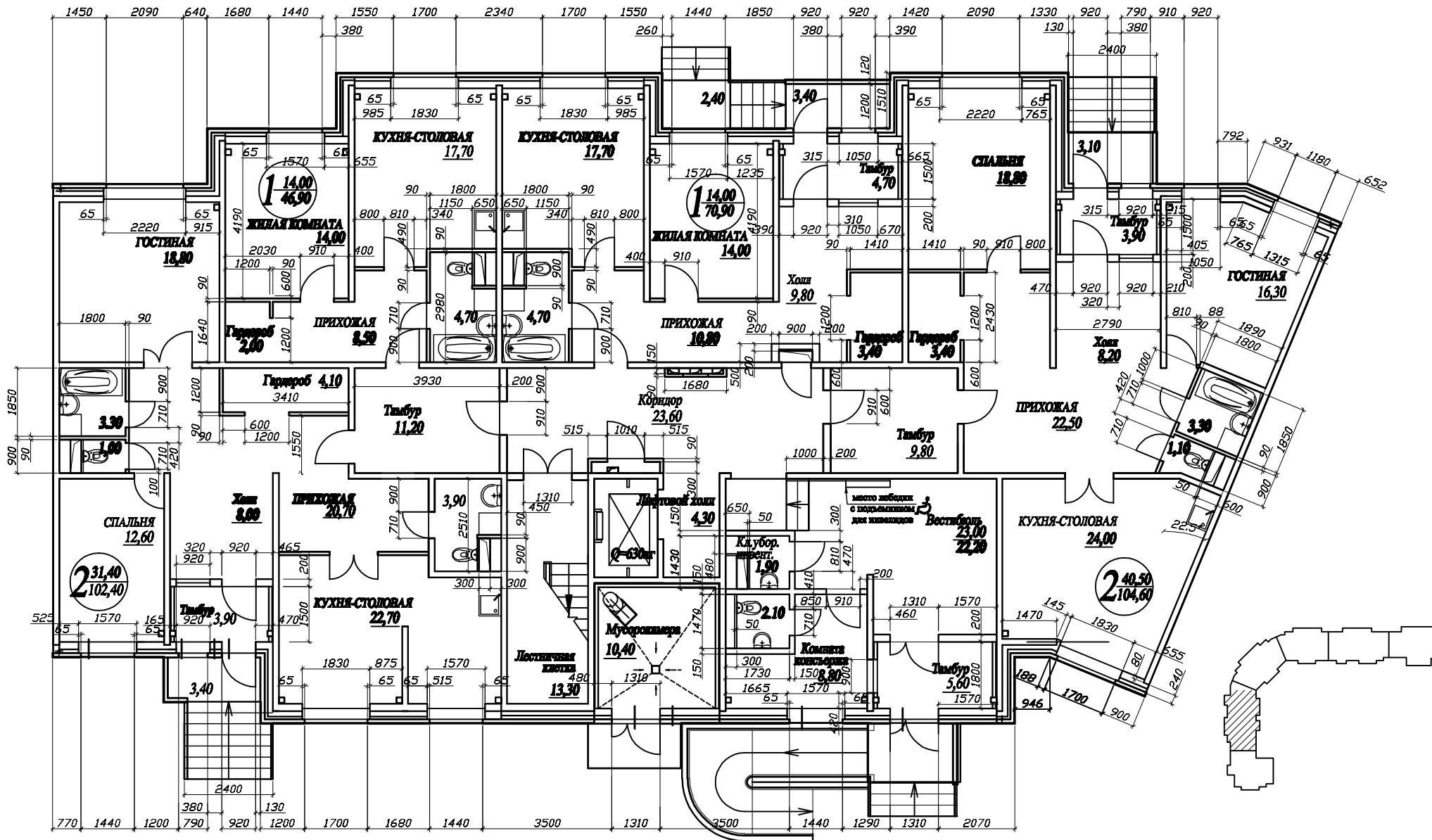
Корпус № 1. Секция 2
