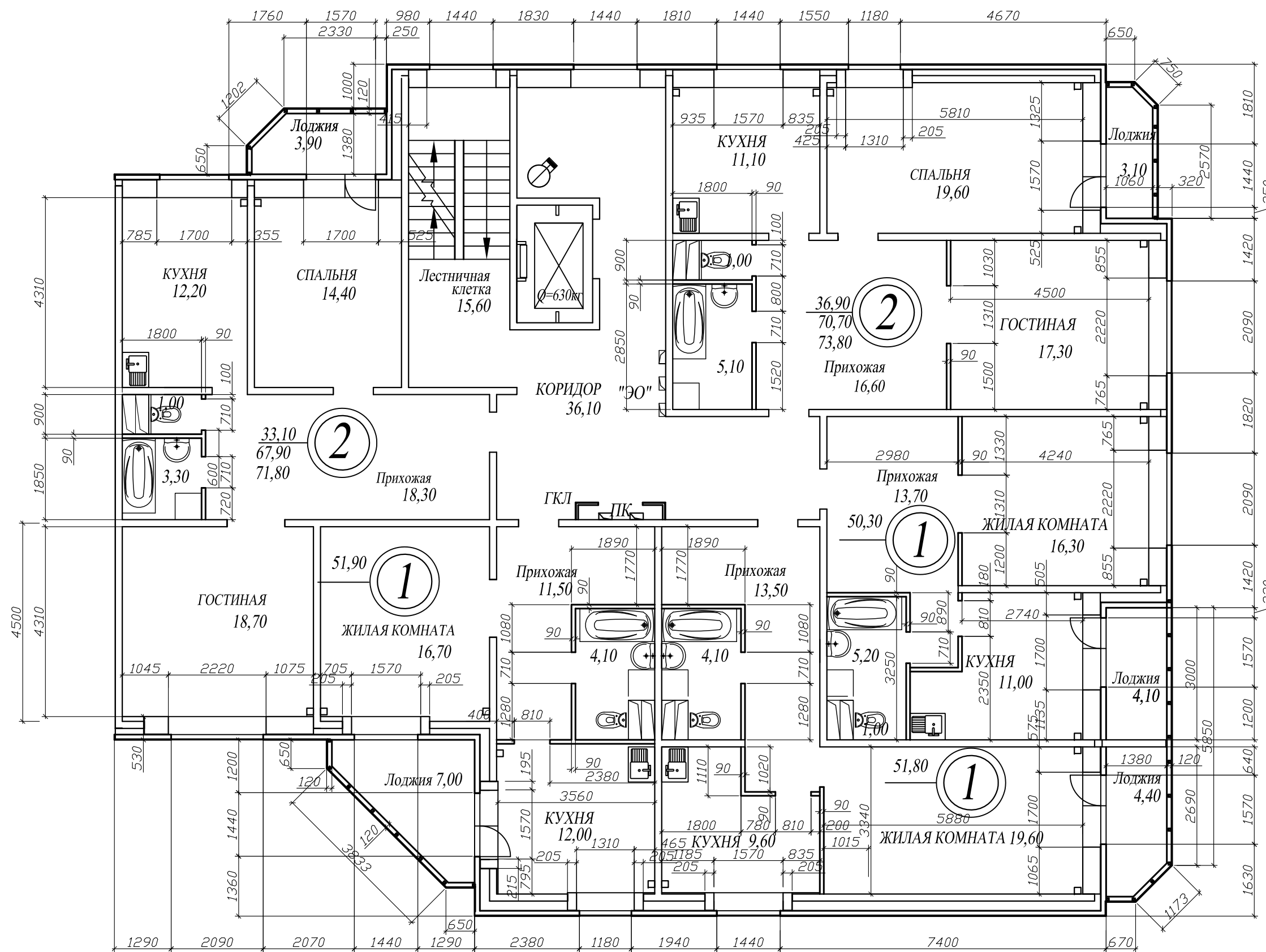
Корпус 16. Секция 7. План 3-7 этажей
