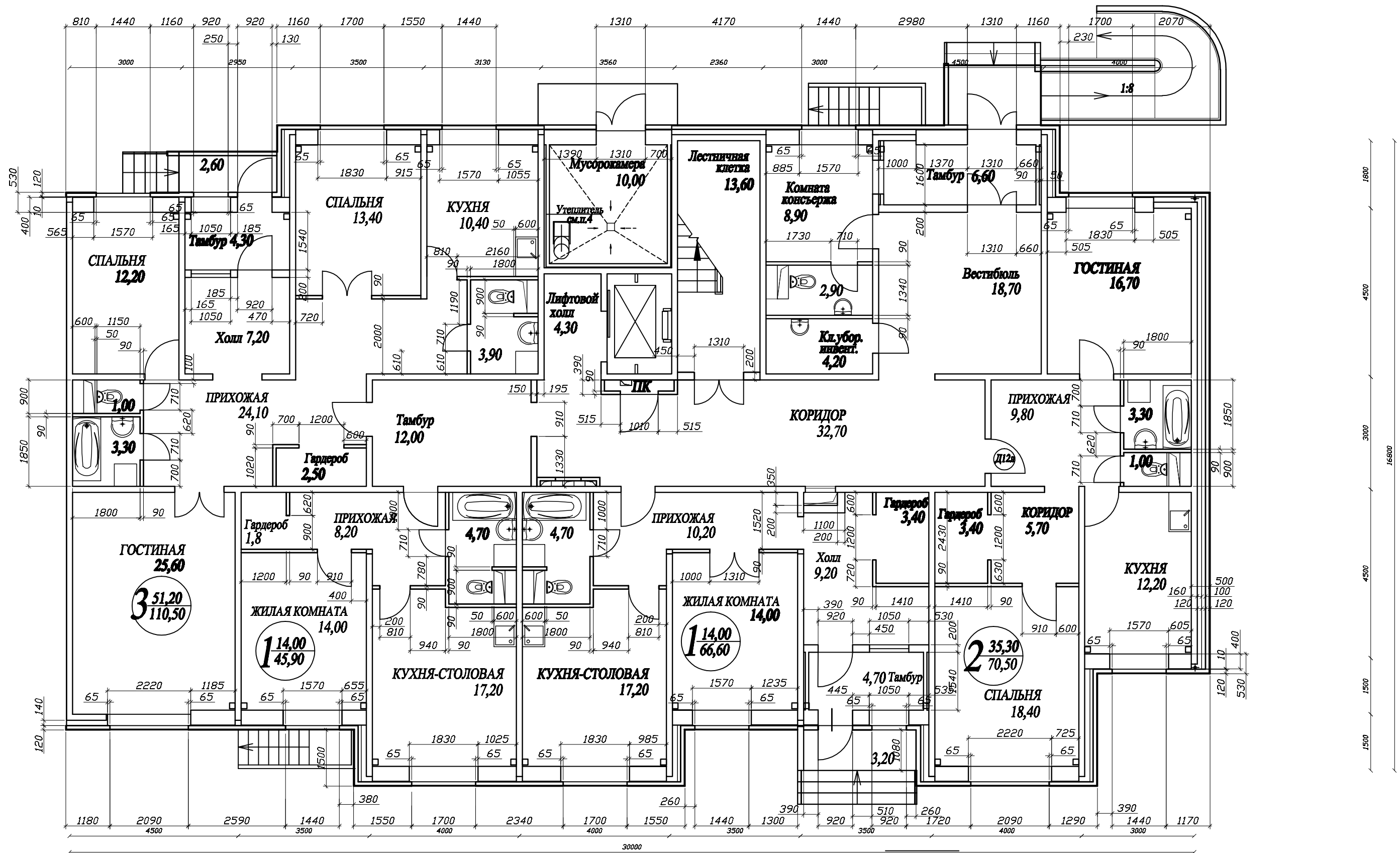
Корпус № 18. Секция 1. План 1 этажа
