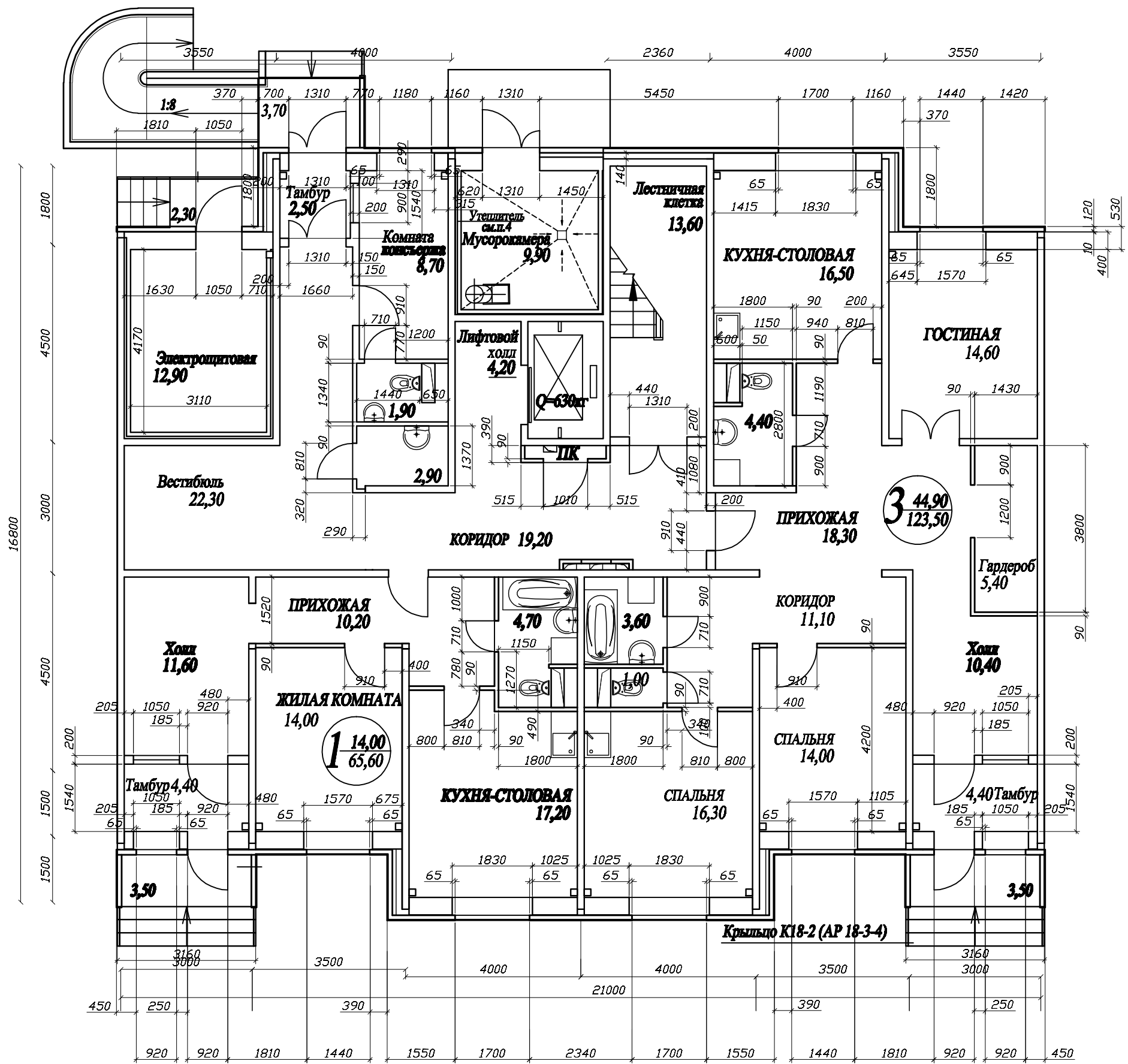
Корпус № 18. Секция 3. План 1 этажа
