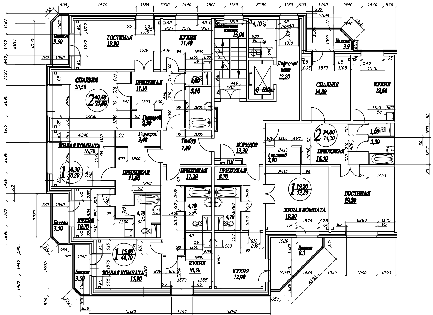
Корпус № 3. Секция 1 План 2-го...9-го этажей
