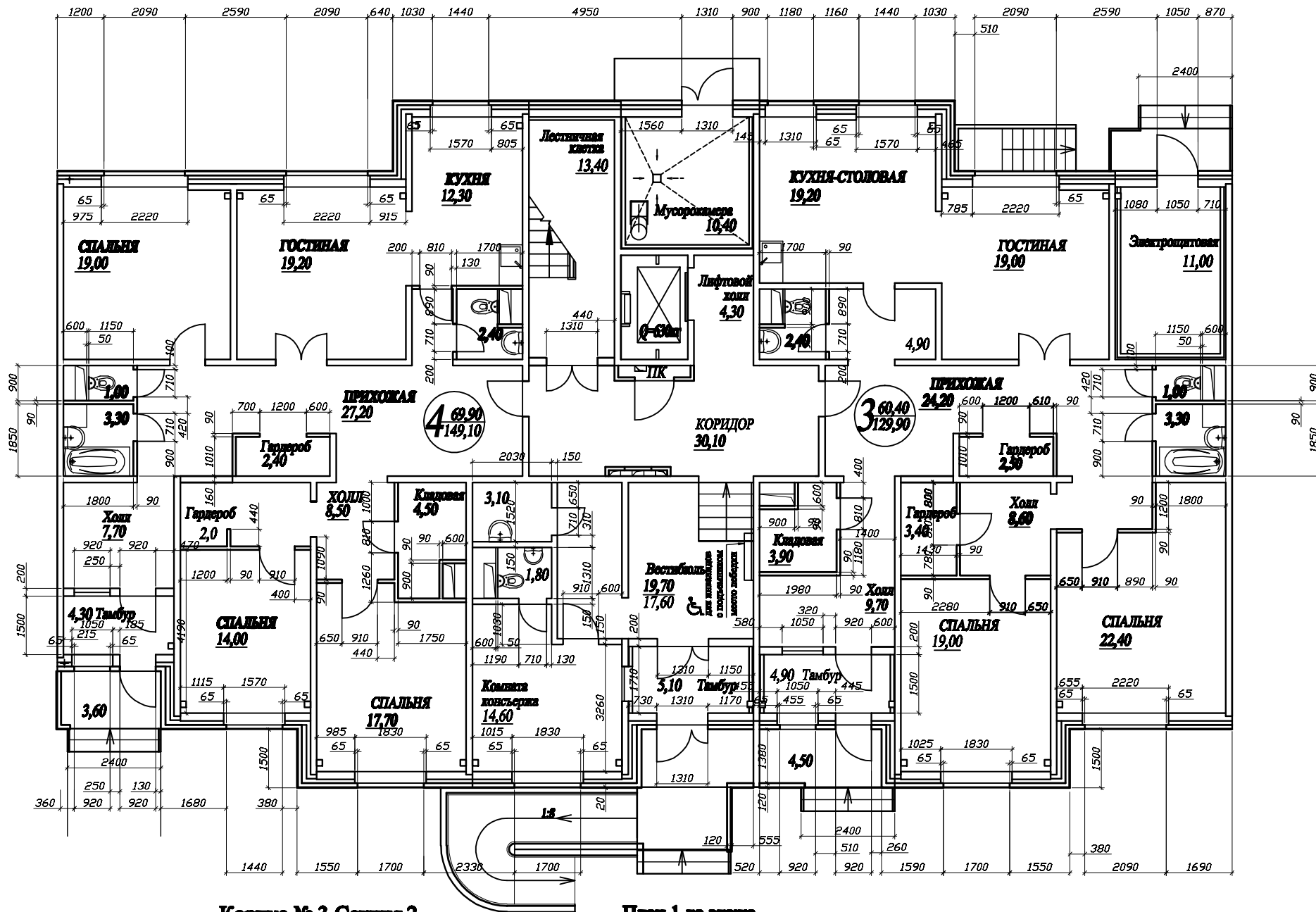
Корпус № 3. Секция 2
