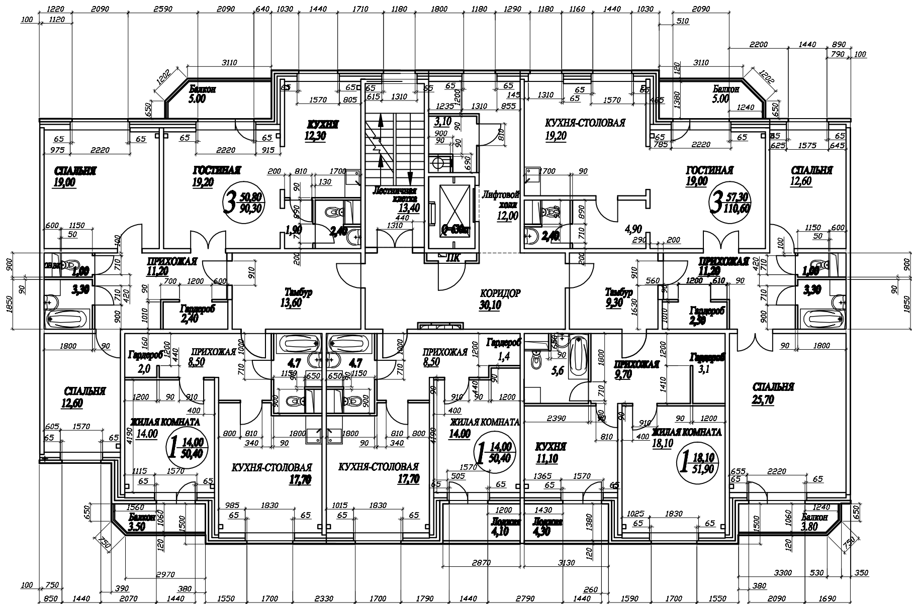
Корпус № 3. Секция 2 Планы 2-го...9-го этажей
