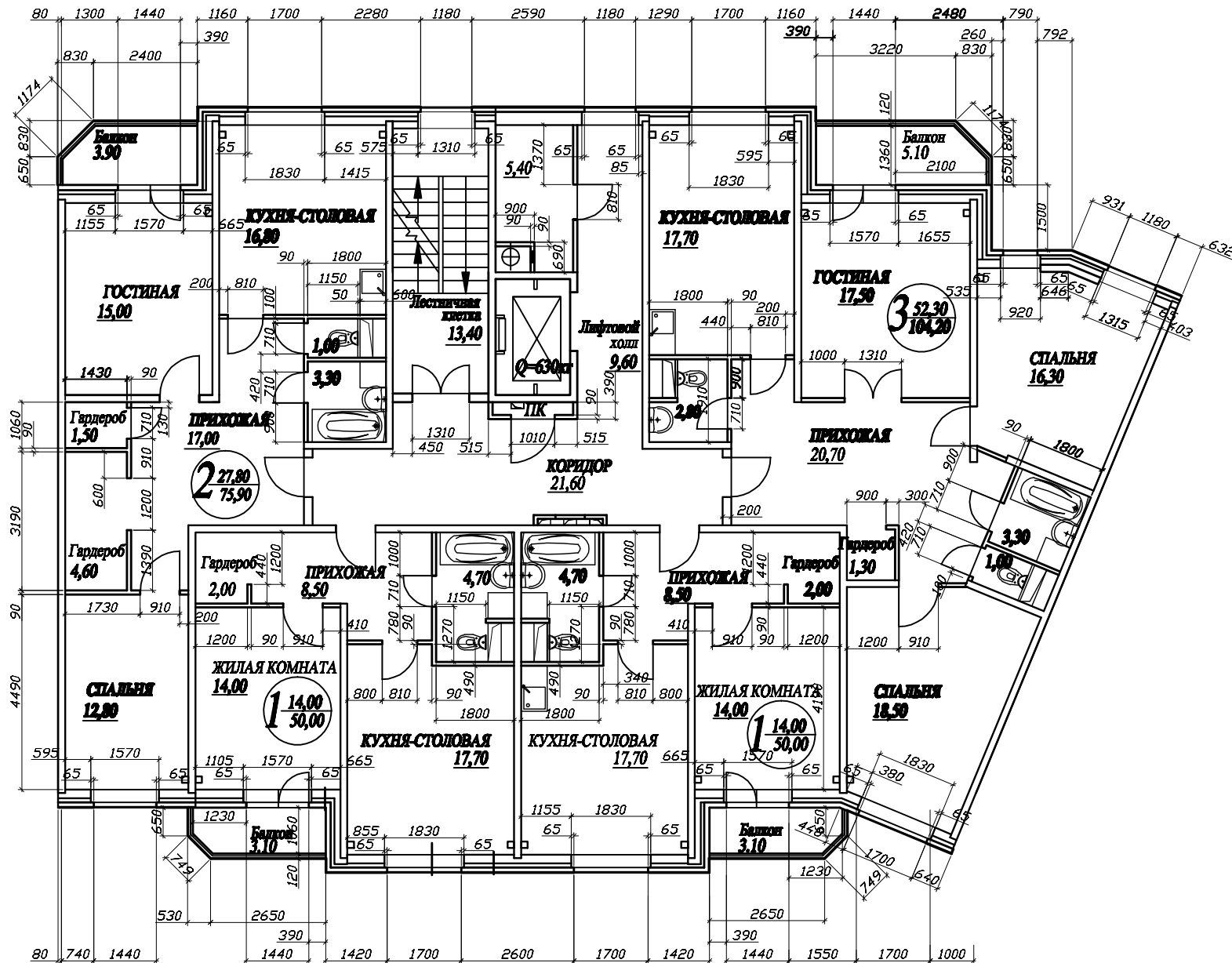
Корпус № 3. Секция 3. Планы 2-го...9-го этажей
